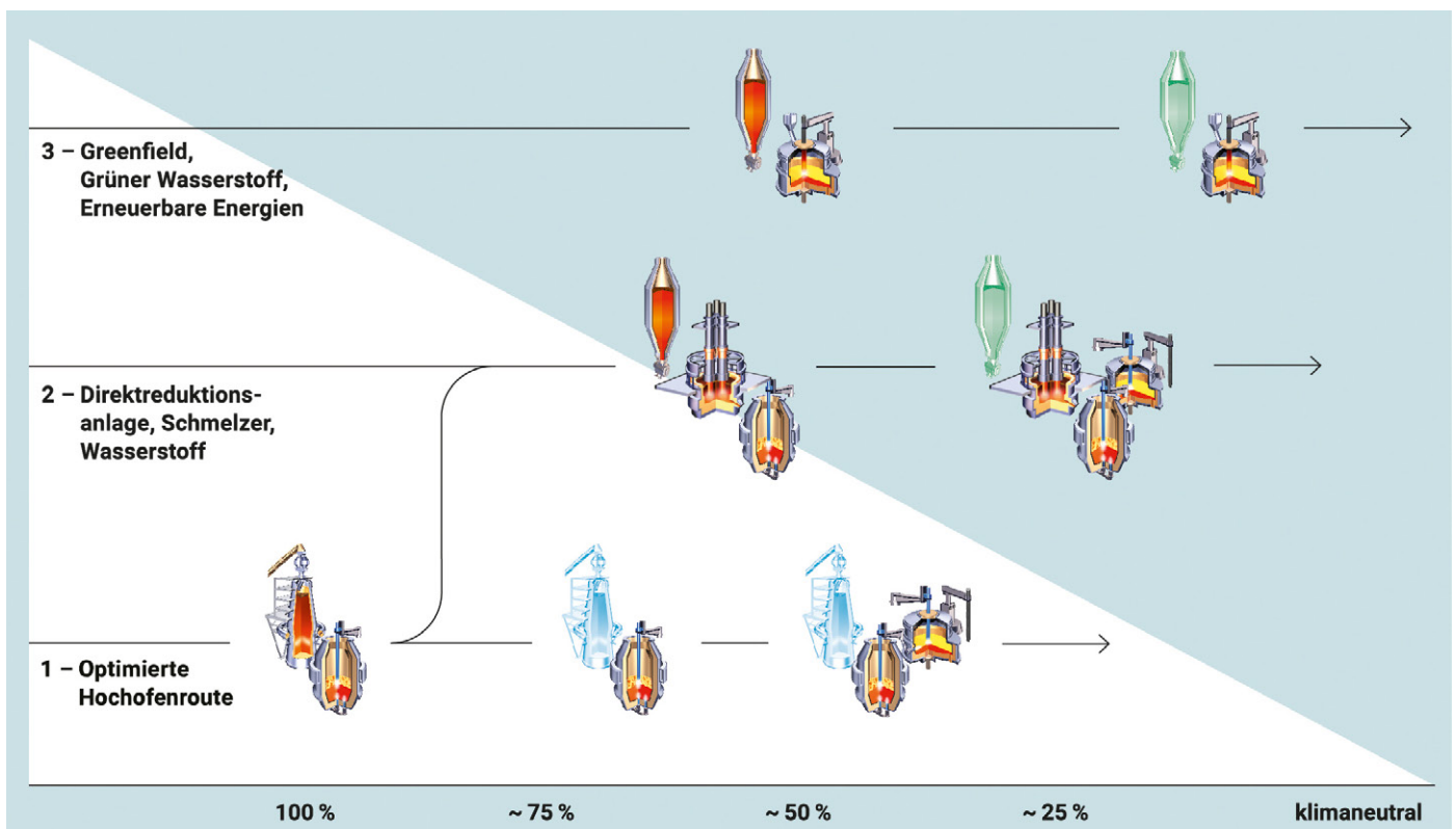
Schematische Darstellung von drei Wegen zur Transformation der Stahlherstellung: Optimierung der Hochofenroute, Integration einer Direktreduktionsanlage in bestehende Hüttenwerke und Neubau von Werken basierend auf grünem Wasserstoff.
