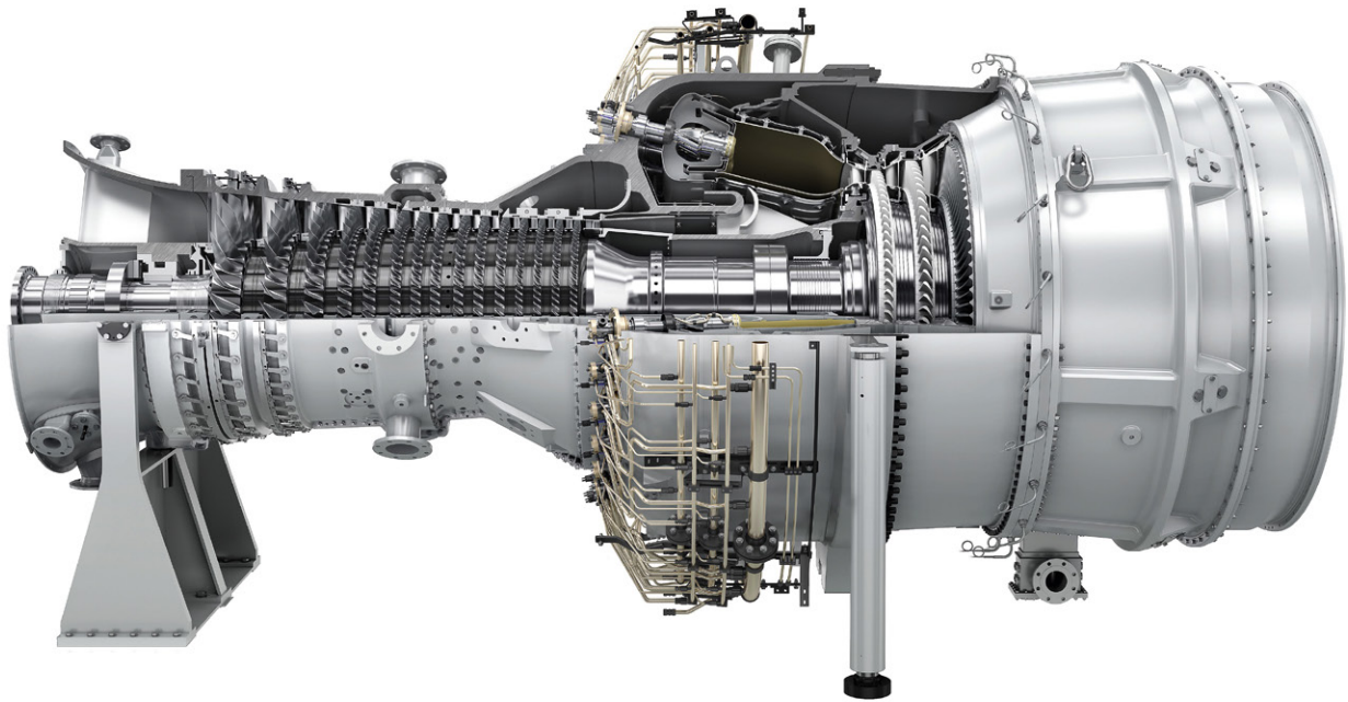
Die im Heizkraftwerk Leipzig Süd zum Einsatz kommenden Gasturbinen sollen ab Ende 2022 mit Erdgas befeuert werden und sukzessive auf die Verbrennung immer größerer Anteile von Wasserstoff umgestellt werden. Langfristig ist ein Betrieb mit 100 Prozent grünem Wasserstoff geplant.
