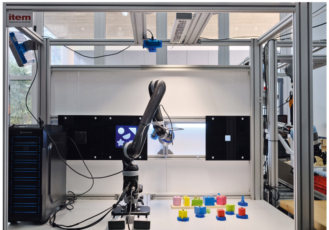
Abbildung 20: Autonomer Fügeprozess mit verschieden geformten Gegenständen.
