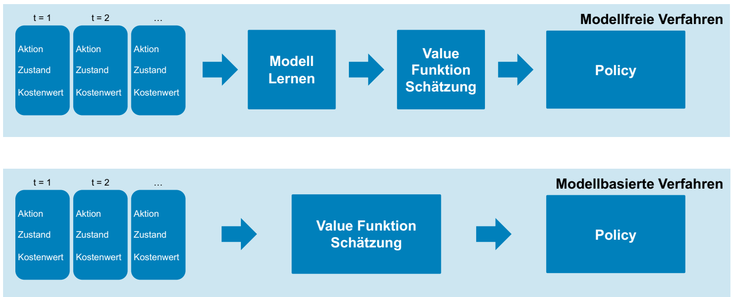
Abbildung 15: Unterschied zwischen modellfreien und modellbasierten Reinforcement Learning Verfahren.
