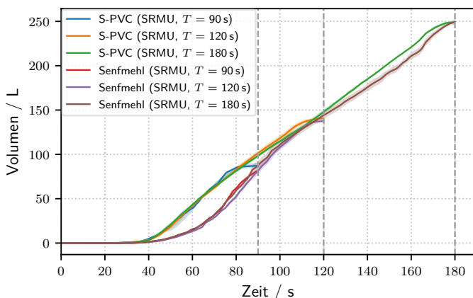
Abbildung 24: Übertragung der Policy für Kunststoffpulver auf Senfmehl. Die blaue Trajektorie zeigt die ursprünglich gelernte Policy für das Kunststoffpulver. Mithilfe dieser Policy wurde dann zunächst über einen längeren Zeitraum von 120 bzw. 180 Sekunden gefördert
