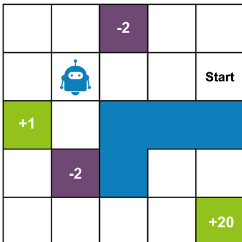
Abbildung 9: diskrete Zustands- und Aktionsräume am Beispiel der so genannten Grid-World.
