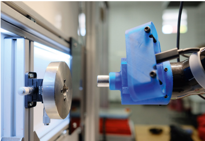
Abbildung 19: Autonomer Montageprozess anhand einer Stift-in-Loch Aufgabe.
