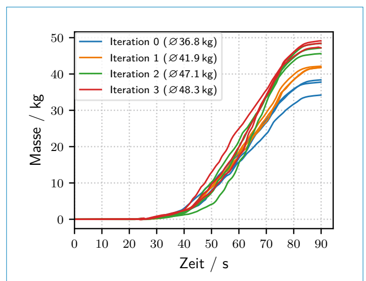
Abbildung 22: Förderung eines Kunststoffgranulats. Die blauen Trajektorien zeigen das Förderverhalten der initial gewählten Policy. Im Laufe des Trainings konnte eine Effizienzsteigerung von 31 % erreicht werden.
