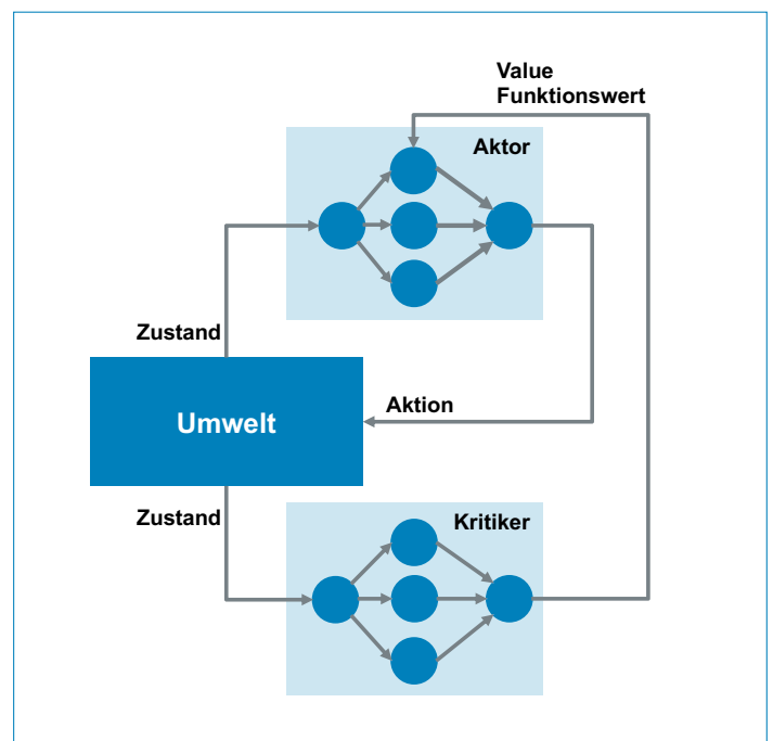
Abbildung 17: Ein Aktor-Kritiker Verfahren besteht aus zwei neuronalen Netzen, welche immer abwechselnd trainiert werden.
