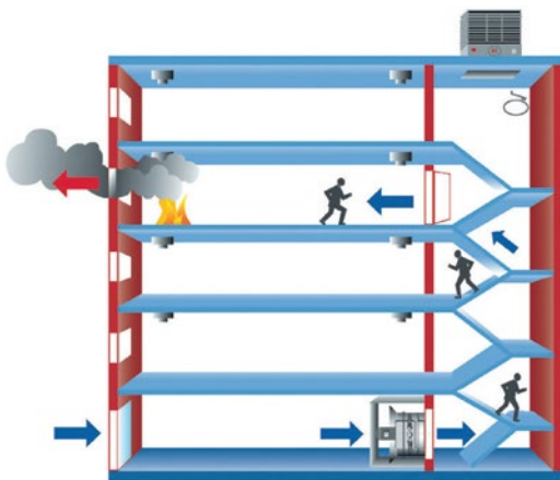
Bild 7: Druckbelüftungsanlagen
